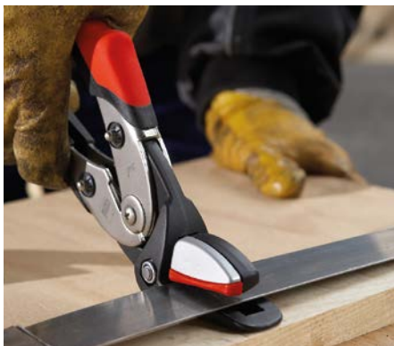
Bandeisen lassen sich mit der Spezialschere schnell und sicher durchtrennen. Dabei wird das Bandeisen beim Schnitt festgehalten.
