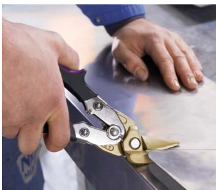
Vor allem bei Edelstahlblechen hat sich der Einsatz von Hochleistungsscheren schon oft bezahlt gemacht.
